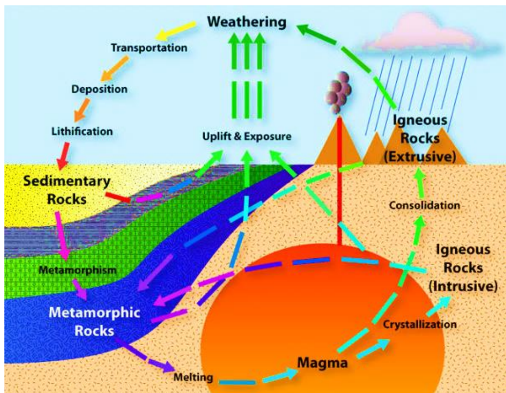
Gambar 2.1 Siklus Batuan
