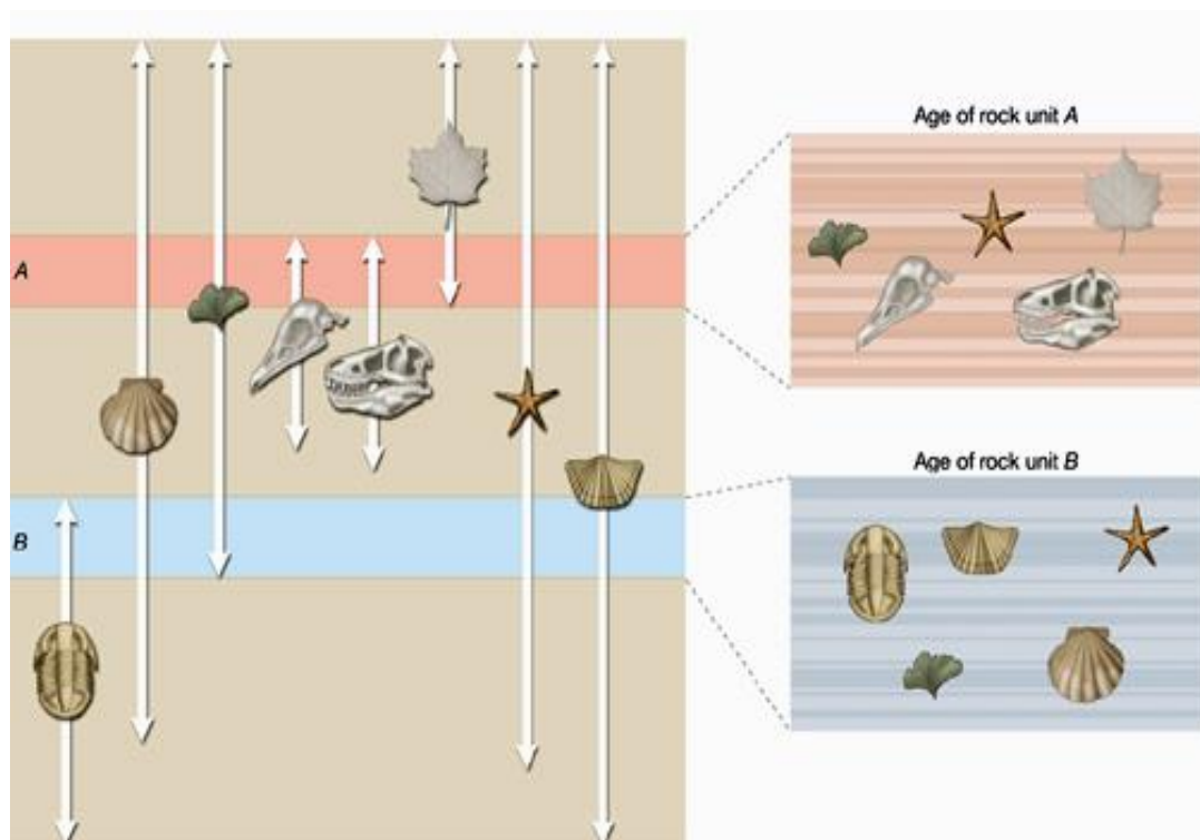
Gambar 5.5 Penentuan umur batuan dilihat dari jenis fosilnya
