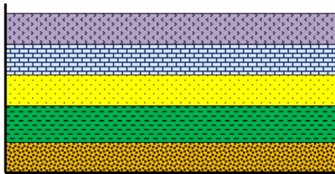
Batuan yang paling tua berada dibawah dan batuan termuda paling atas
