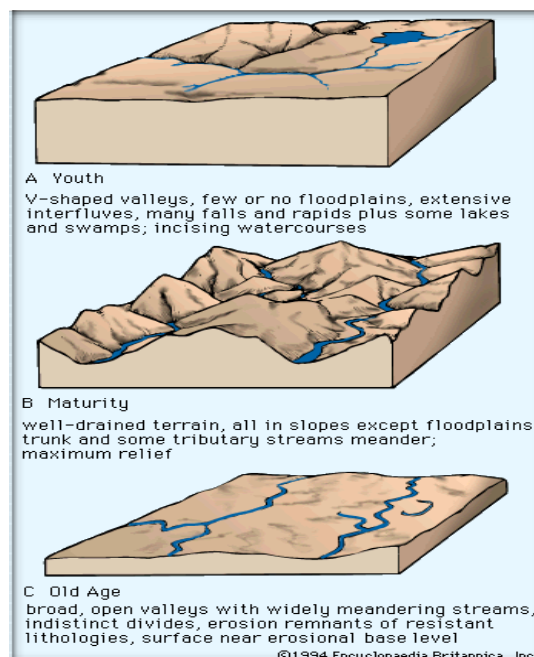
Gambar 5.1 Stadia muda, dewasa dan tua. (sumber : http://media-3.web.britannica.com/eb-media/55/7755-004-A569A5BA.gif )
